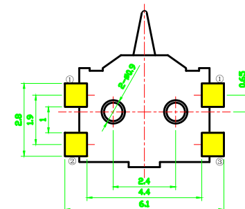
安裝位置圖
