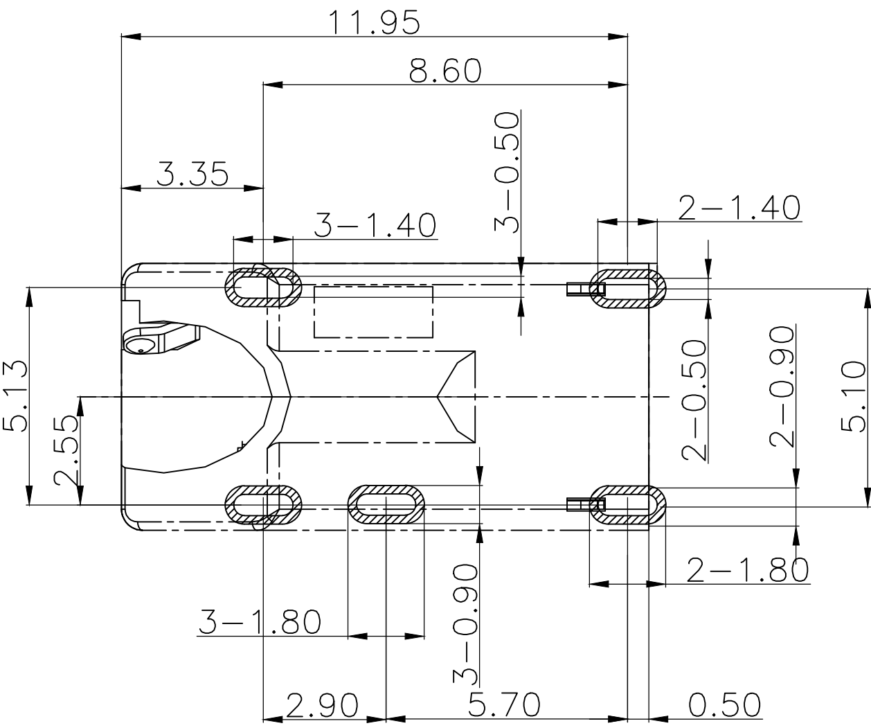
P.C.B LAYOUT
