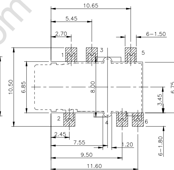
P.C.B LAYOUT TOP VIEW 反贴
