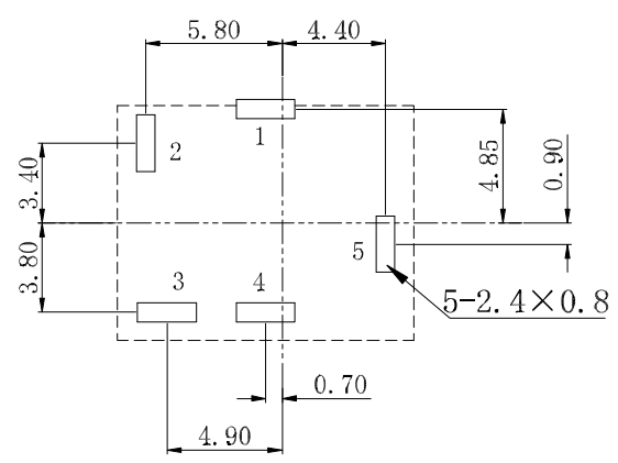
线路板开孔尺寸
