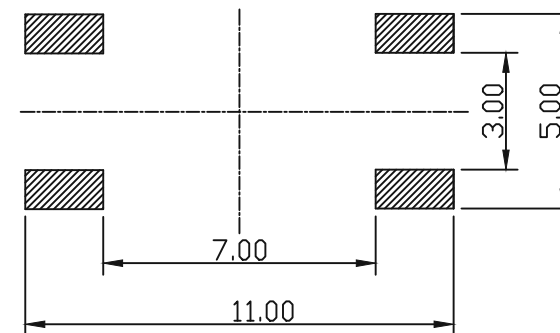
PCB. 焊接图
