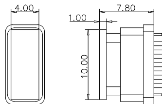
装前塞示意图
