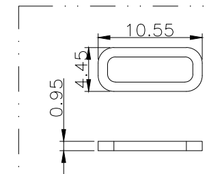
防水圈图示
