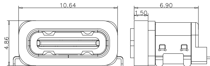
加防水圈示意图
