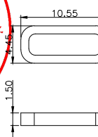
防水圈图示
