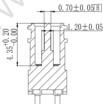
截面A-A
