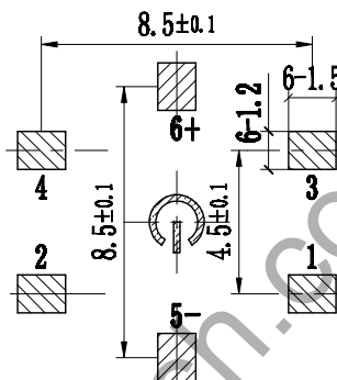
元件面孔位图
