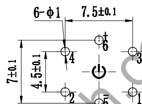
元件面孔位图
